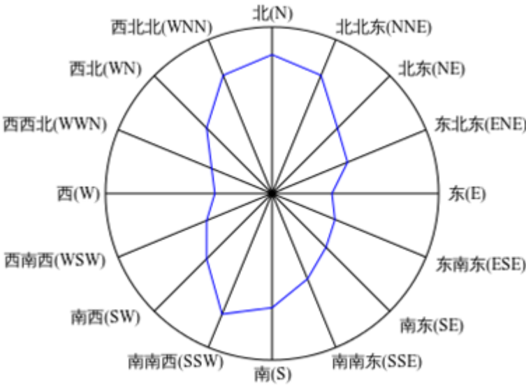
图 3.18.1-1 风向玫瑰图
