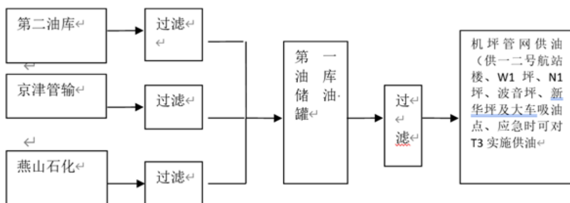
图 2.2-1 工艺流程图
